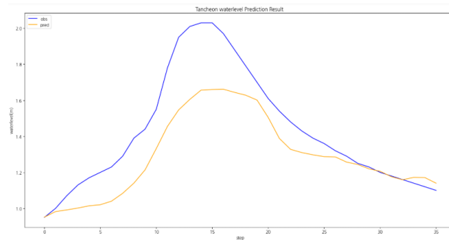
testdata_250716
