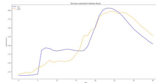
05_mae
