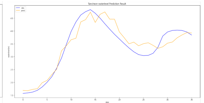
testdata_220808
