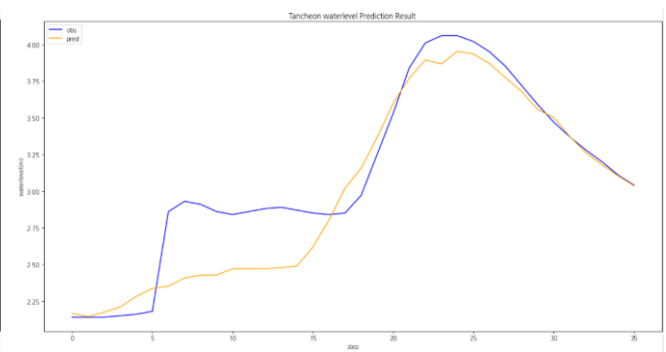
testdata_250814
