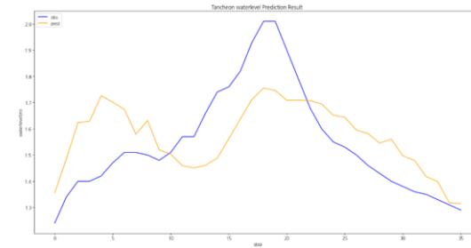
06_mse
