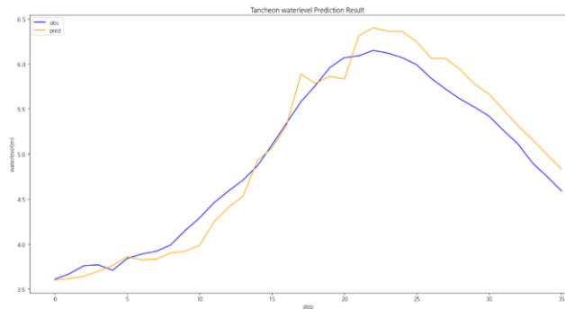
testdata_220630 (mae)
