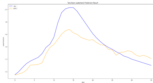
testdata_250716
