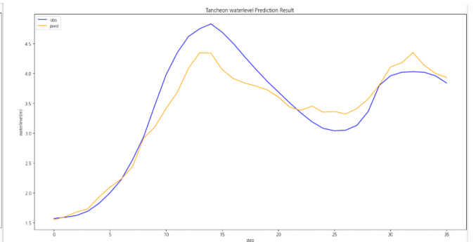
testdata_220808
