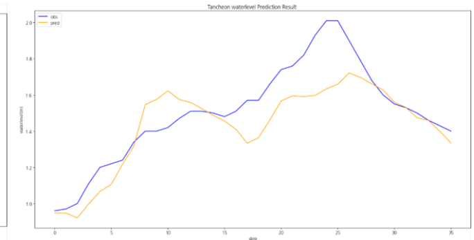
testdata_250814
