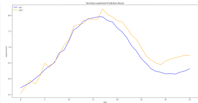
testdata_220808 (mae)
