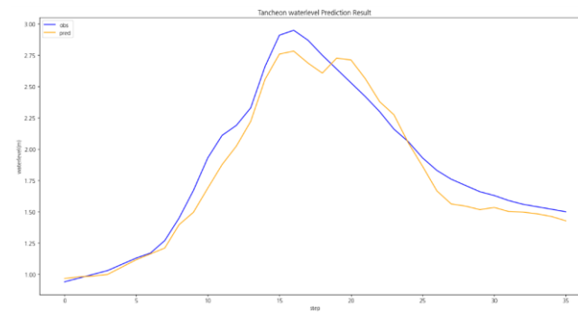
testdata_170723
