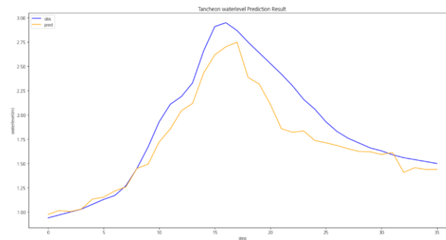
testdata_170723
