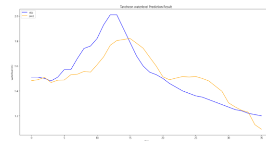
07_mse
