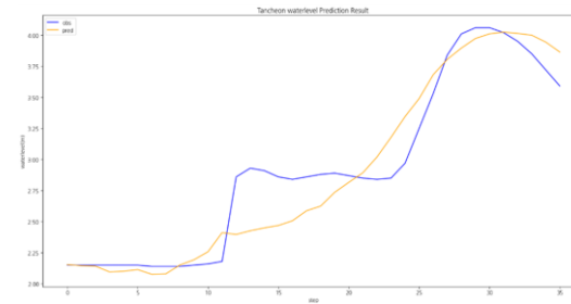
04_mae
